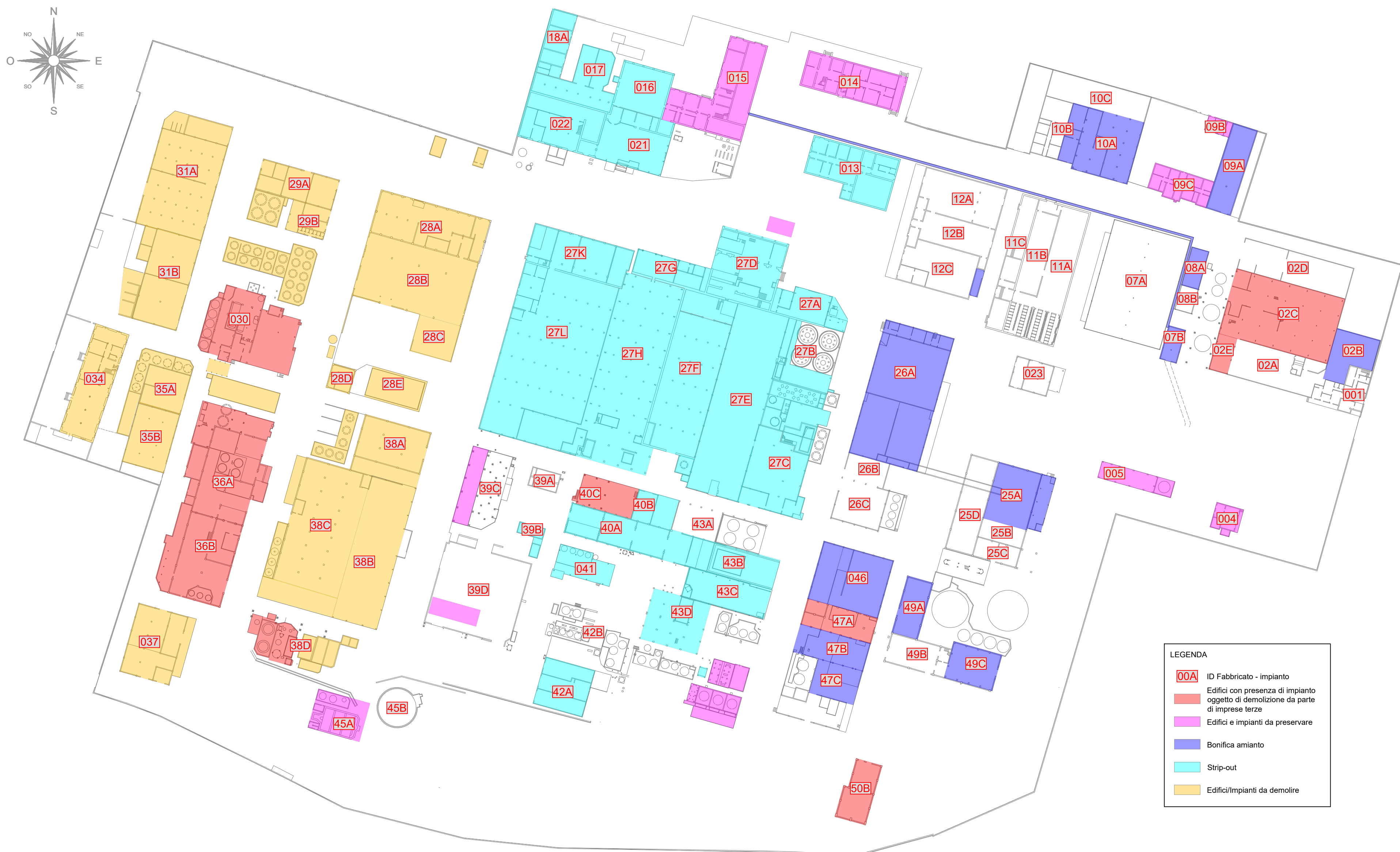
FASE D: Bonifica di MCA presenti negli edifici di Fase 4 del progetto definitivo (ove presente), proseguimento strip-out degli edifici di Fase 3 del progetto definitivo (ove presente) e demolizione degli edifici di Fase 2 del progetto definitivo - 1:1000
